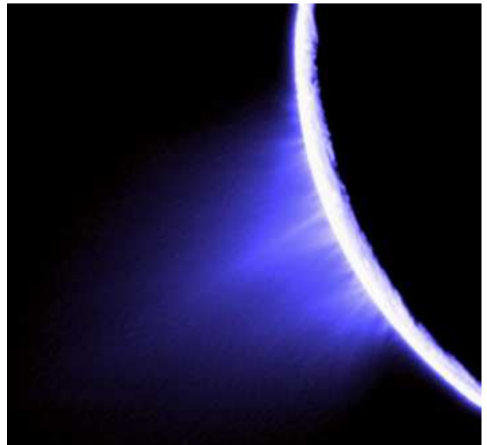
Bức ảnh này do tàu thăm dò Cassini gửi về ngày 27-11-2005 cho thấy dấu hiệu về sự tồn tại của nước trên vệ tinh Enceladus của sao Thổ. Hơi nước và tinh thể băng thoát ra từ Enceladus tạo thành những cột mây khổng lồ có chiều cao gần 150.000km
