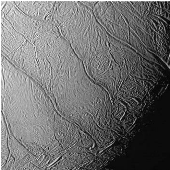
Cận cảnh những đường đứt gãy song song gồ ghề tựa như những sọc vằn trên da hổ (Tiger Stripes) được chụp ngày 14-7-2005 ở độ vĩ Nam của Enceladus - vệ tinh lớn thứ sáu của sao Thổ
