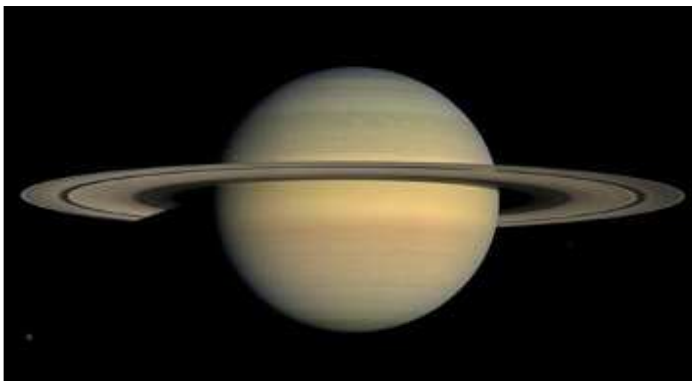
Toàn cảnh sao Thổ do tàu Cassini chụp với góc độ rộng ngày 23-7-2008
