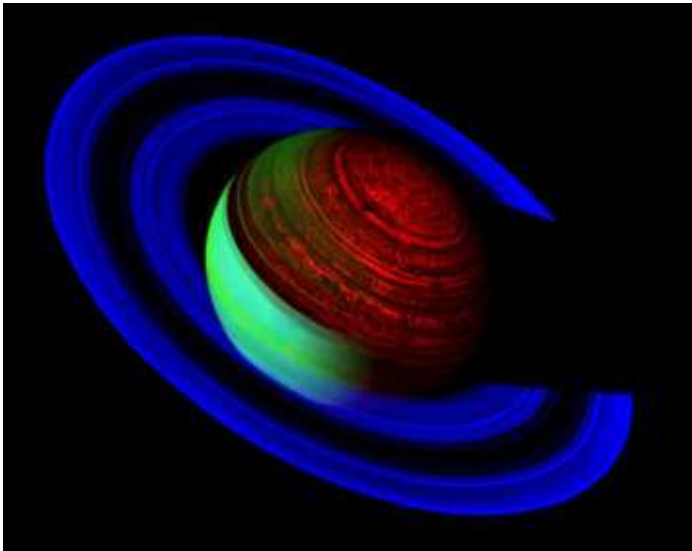
Những khám màu giả đầy ấn tượng vòng quanh sao Thổ được các nhà khoa học kết hợp từ 25 bức ảnh do phi thuyền Cassini chụp ngày 24-2-2007
