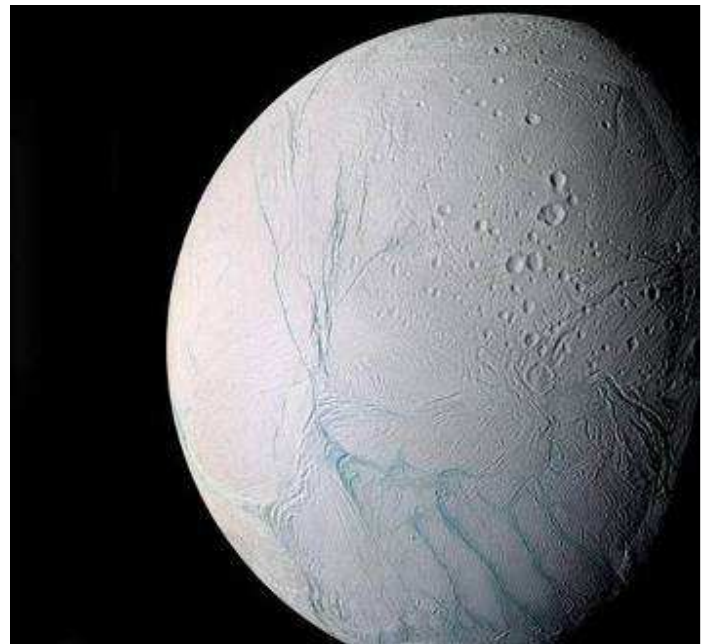
Những đường đứt gãy địa chất màu xanh trên Enceladus được bao quanh bởi những miệng núi lửa cổ xưa trên vệ tinh Enceladus sao Thổ do phi thuyền Cassini-Huygens chụp được trong khoảng thời gian từ 9-3 đến 14-7-2005
