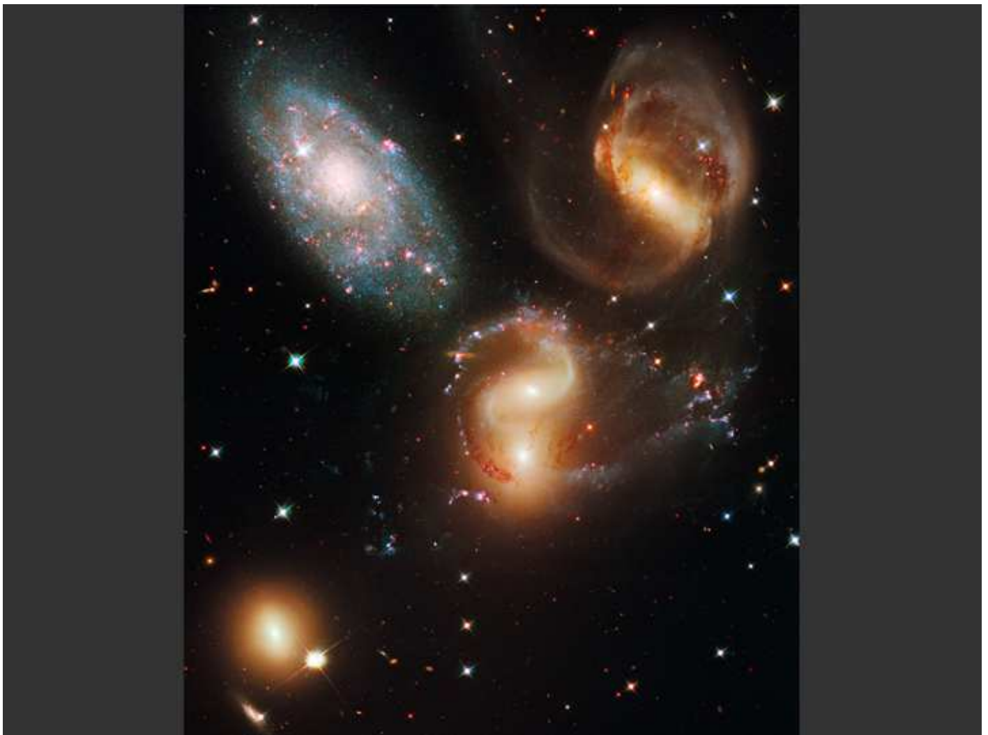
Le « Quintet de Stephan »
