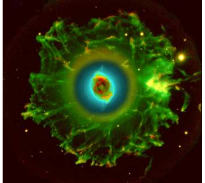
Chat (..... OUI, un chat du nom NGC 6543)
